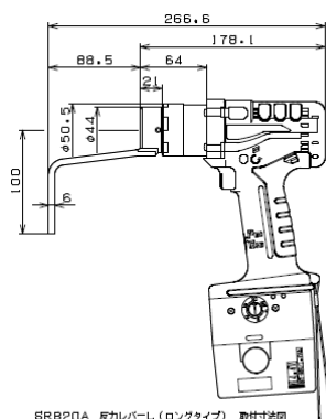
SRB20A 反力レバーL (ロングタイプ) 取付寸法図 H2D/11/06 印刷
