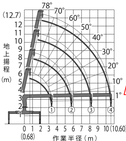
大型クレーン4段 (URG504S)
