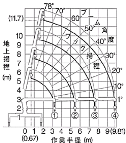
標準クレーン4段 (URG344N)
